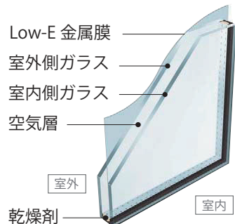
Low-E複層ガラス
